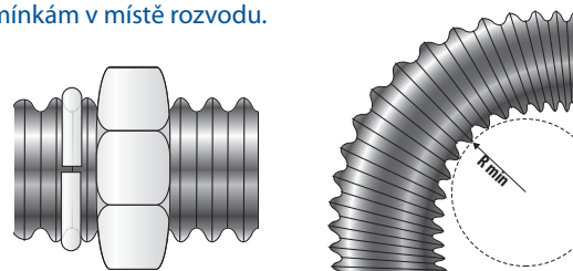
správné umístění nerezového půleného upevňovacího kroužku
