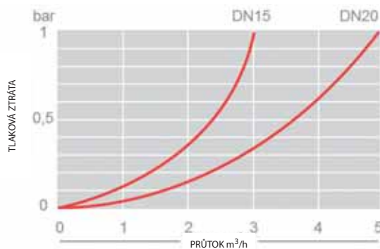
Diagram tlakových ztrát vodoměrů DN 15 a DN 20
