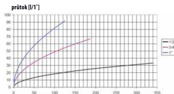
DIAGRAM TLAKOVÝCH ZTRÁT (40% ROZTOK GLYKOLU PŘI 40 °C)
