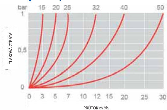
Diagram tlakových ztrát vodoměrů od DN 15 do DN 50
