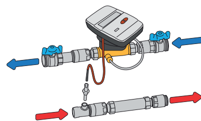
Obvyklý způsob instalace měřiče tepla na zpátečku.
